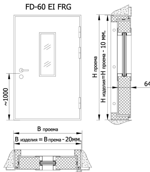
Вариант исполнения полотна
