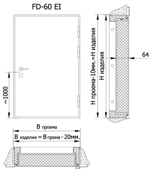
Варианты крепления рамы к проему
