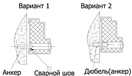
Варианты крепления рамы к проему
